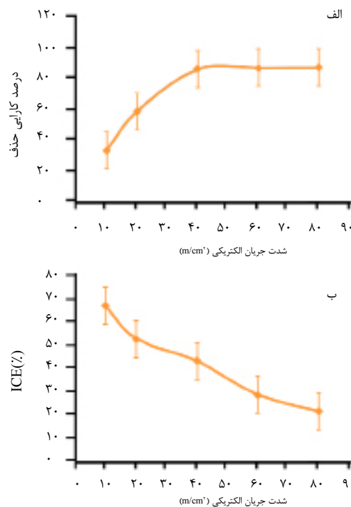
نمودار ۴. الف) تأثیر تغییرات شدت جریان الکتریکی در تصفیه فاضلاب کارخانه کاشمش پاک کنی و (ب) کارایی انرژی لحظه ای (ICE)، در شرایط ثابت \text{pH}=3 و مدت زمان ماند 360 \text{ min} طی فرآیند الکترواکسیداسیون
