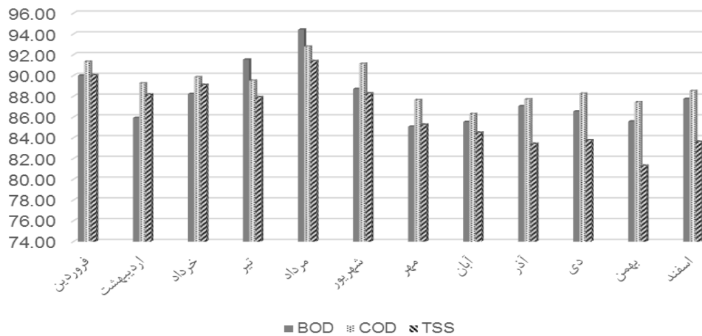
شکل ۲: نمودار مقایسه‌ای راندمان حذف BOD, COD و TSS تصفیه خانه فاضلاب بجنورد
