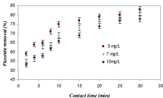
نمودار ۳: تاثیر غلظت فلوراید و زمان تماس در فرایند جذب (pH برابر ۷، دوز جاذب ۰،۵ گرم)
