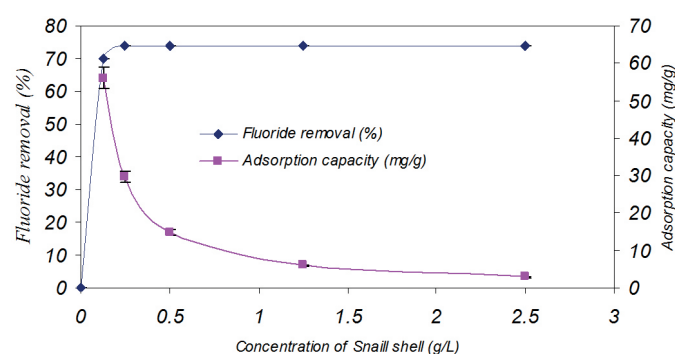
نمودار ۴: تاثیر دز پوسته حلزون در فرایند جذب (غلظت اولیه فلوراید ۱۰ میلی گرم در لیتر، pH برابر ۷، زمان تماس ۳۰ دقیقه)
