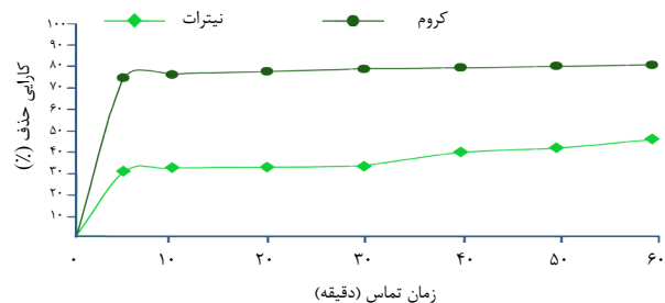
نمودار ۴. تاثیر زمان تماس بر کارایی حذف همزمان کروم (VI) و نیترات (مقدار فلز منیزیم ۰/۱۷ g/L، دمای ۲۵°C، غلظت اولیه کروم و نیترات ۱۰۰ میلی گرم در لیتر)
