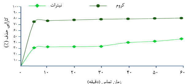
نمودار ۴. تاثیر زمان تماس بر کارایی حذف همزمان کروم (VI) و نیترات (مقدار فلز منیزیم ۰/۷ g/L، دمای ۲۵°C، pH=۳، غلظت اولیه کروم و نیترات ۱۰۰ میلی گرم در لیتر)
