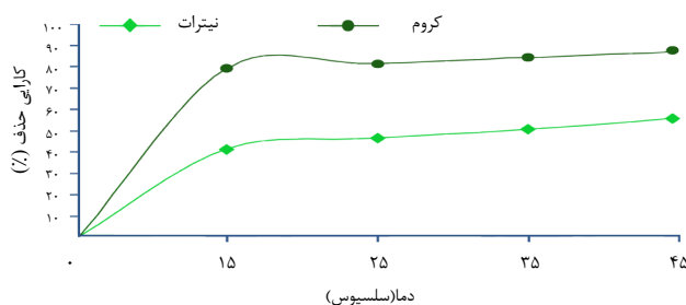
نمودار ۵. تاثیر دما بر کارایی حذف همزمان کروم (VI) و نیترات (مقدار فلز منیزیم ۰/۷ g/L، دمای ۲۵°C، pH=۳، غلظت اولیه کروم و نیترات ۱۰۰ میلی گرم در لیتر)
