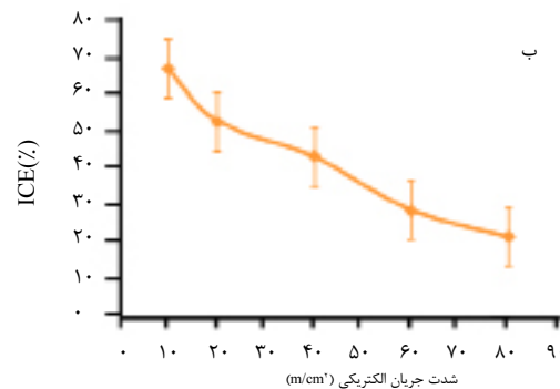
نمودار ۴. الف) تأثیر تغییرات شدت جریان الکتریکی در تصفیه فاضلاب کارخانه کاشمش پاک کنی و (ب) کارایی انرژی لحظه ای (ICE)، در شرایط ثابت \text{pH}=3 و مدت زمان ماند ۳۶۰ min طی فرآیند الکترواکسیداسیون
