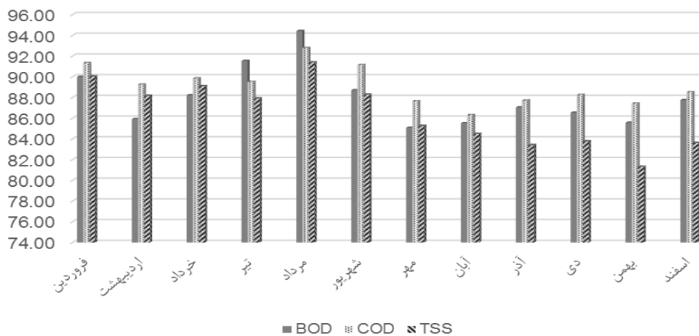
شکل ۲: نمودار مقایسه‌ای راندمان حذف BOD, COD, TSS تصفیه خانه فاضلاب بجنورد
