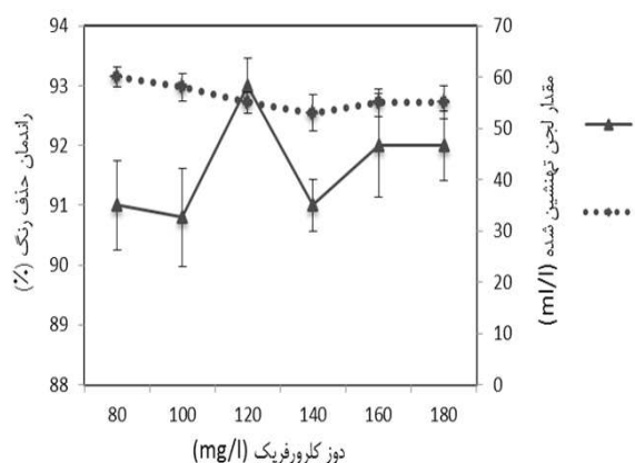
شکل ۴. راندمان حذف و مقدار لجن ته‌نشین شده رنگ دیسپرس آبی توسط فرایند انعقاد در دوز متفاوت آلوم
