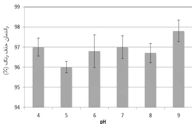
شکل ۳. راندمان حذف رنگ دیسپرس آبی توسط فرایند انعقاد با کلوروفریک در pH متفاوت
